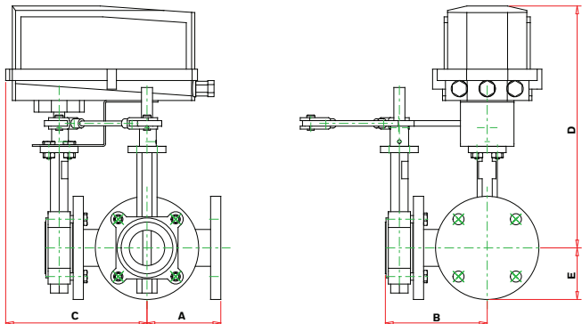
Fig. 12. Vannes à 3 voies avec actionneurs NEMA 2 MBS...1, 3
