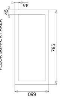
SUPERFICIE PER APOGGIO PLENUM PLENUM SUPPORT AREA
